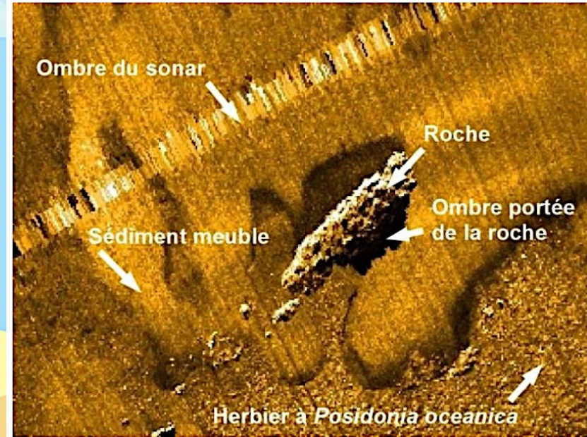
Interprétation d'une image sonar sur un fond marin de Méditerranée (Corse). Source : Arnaud Abadie.
