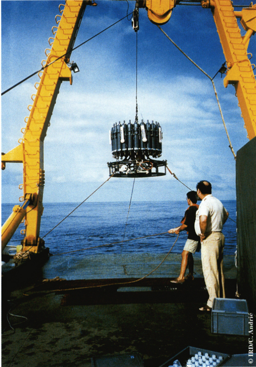
Bathysonde et rosette composée de bouteilles à renversement pour les prélèvements d'eaux en profondeur. Campagne Orstom.
