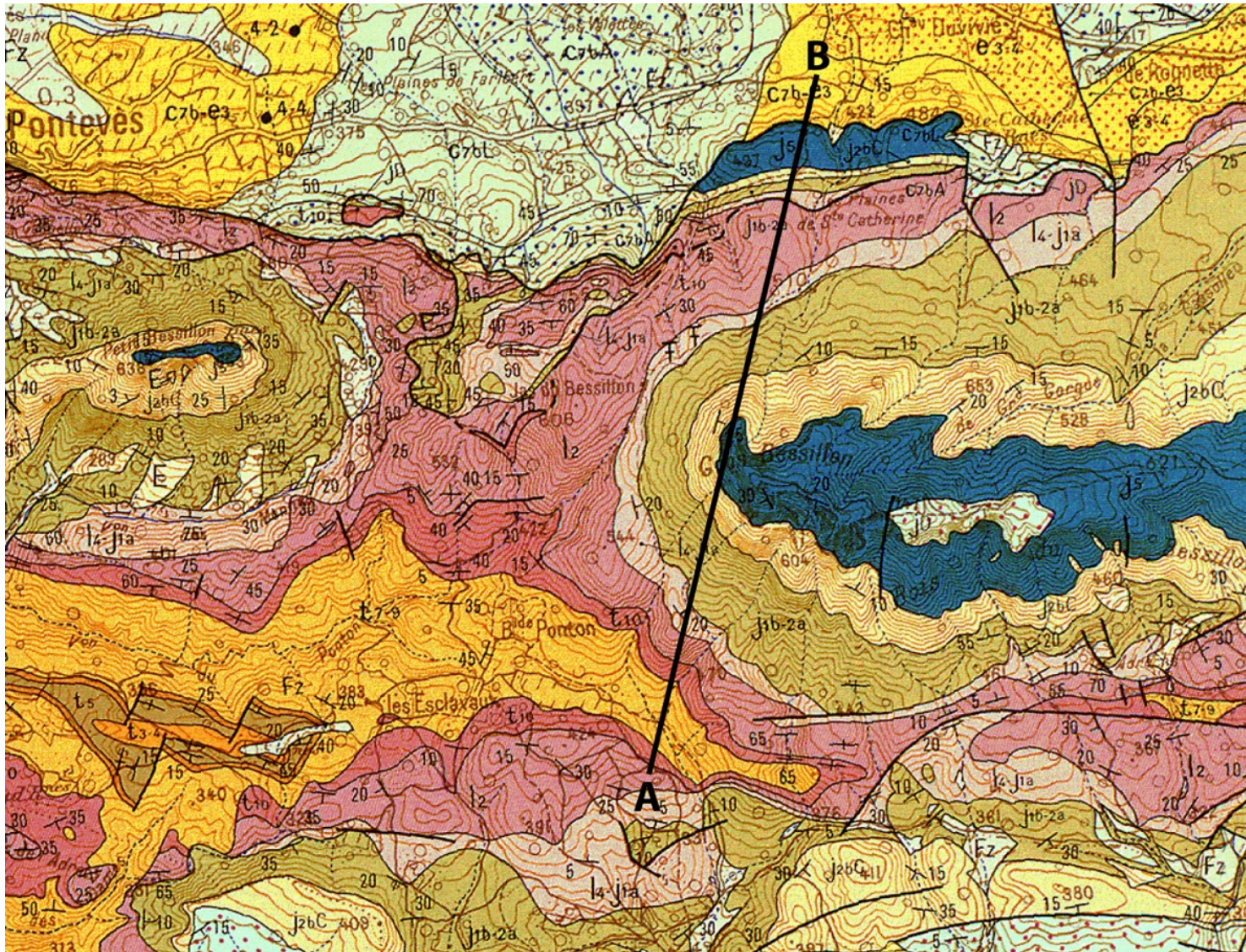
Document 4.c : Extrait de la carte géologique de Brignoles initialement au 50 000 ème . (Source : BRGM)
